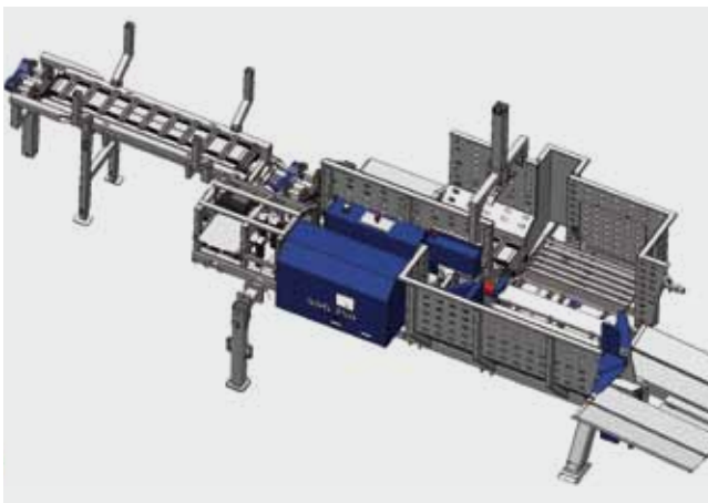
Säge- und Spaltgigant, 3D-Modell
